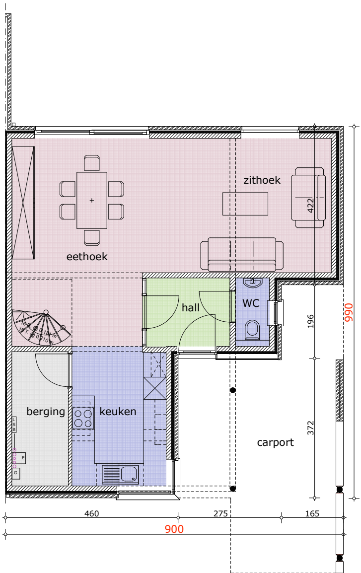
GELIJKVLOERS woning 4-8
