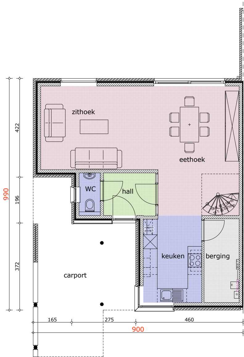
GELIJKVLOERS woning 1-5
