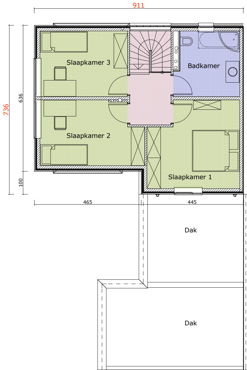
VERDIEPING woning 12 en 20
