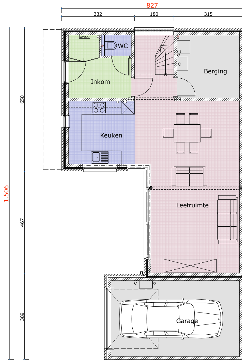
GELIJKVLOERS woning 12 en 20
