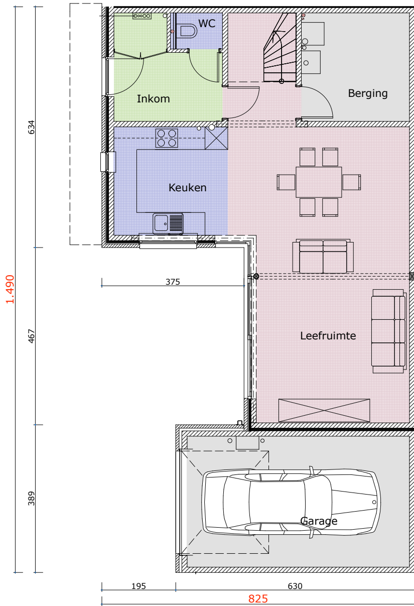
GELIJKVLOERS woning 10 en 18
