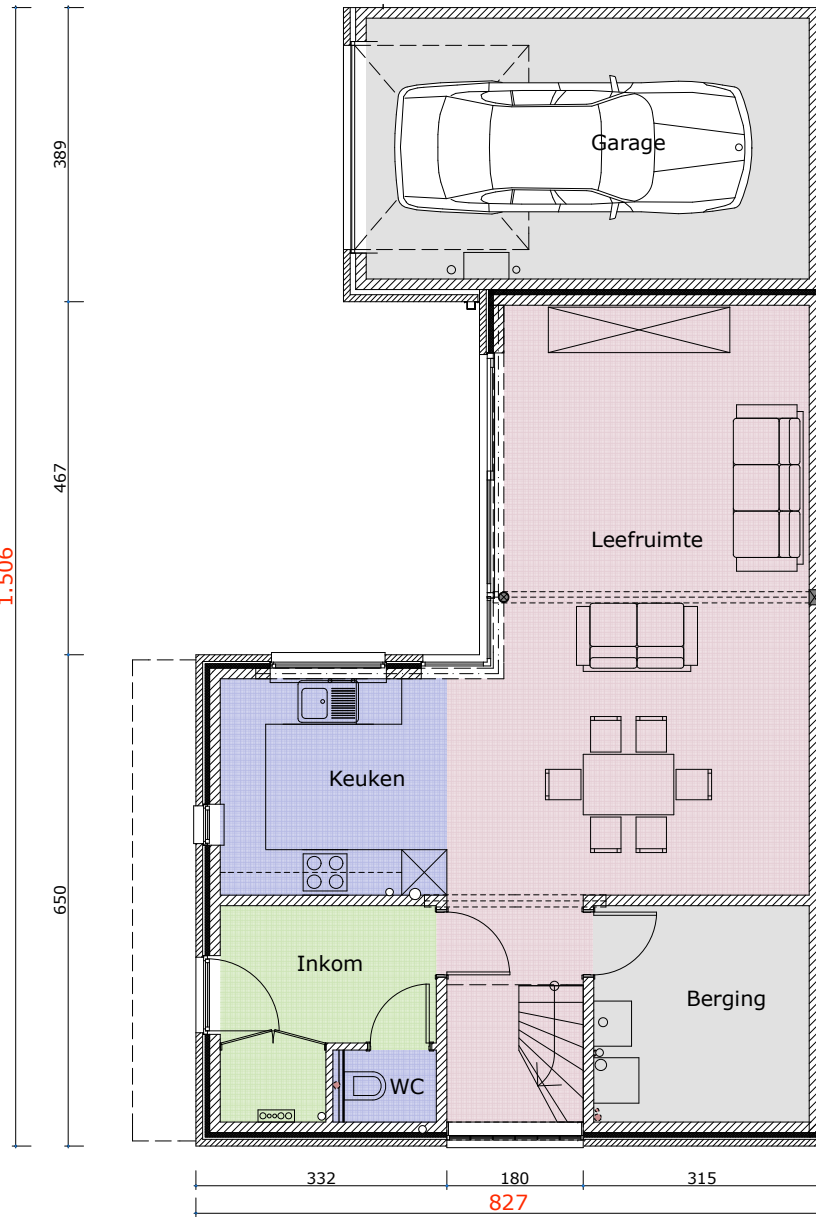
GELIJKVLOERS woning 9 en 17
